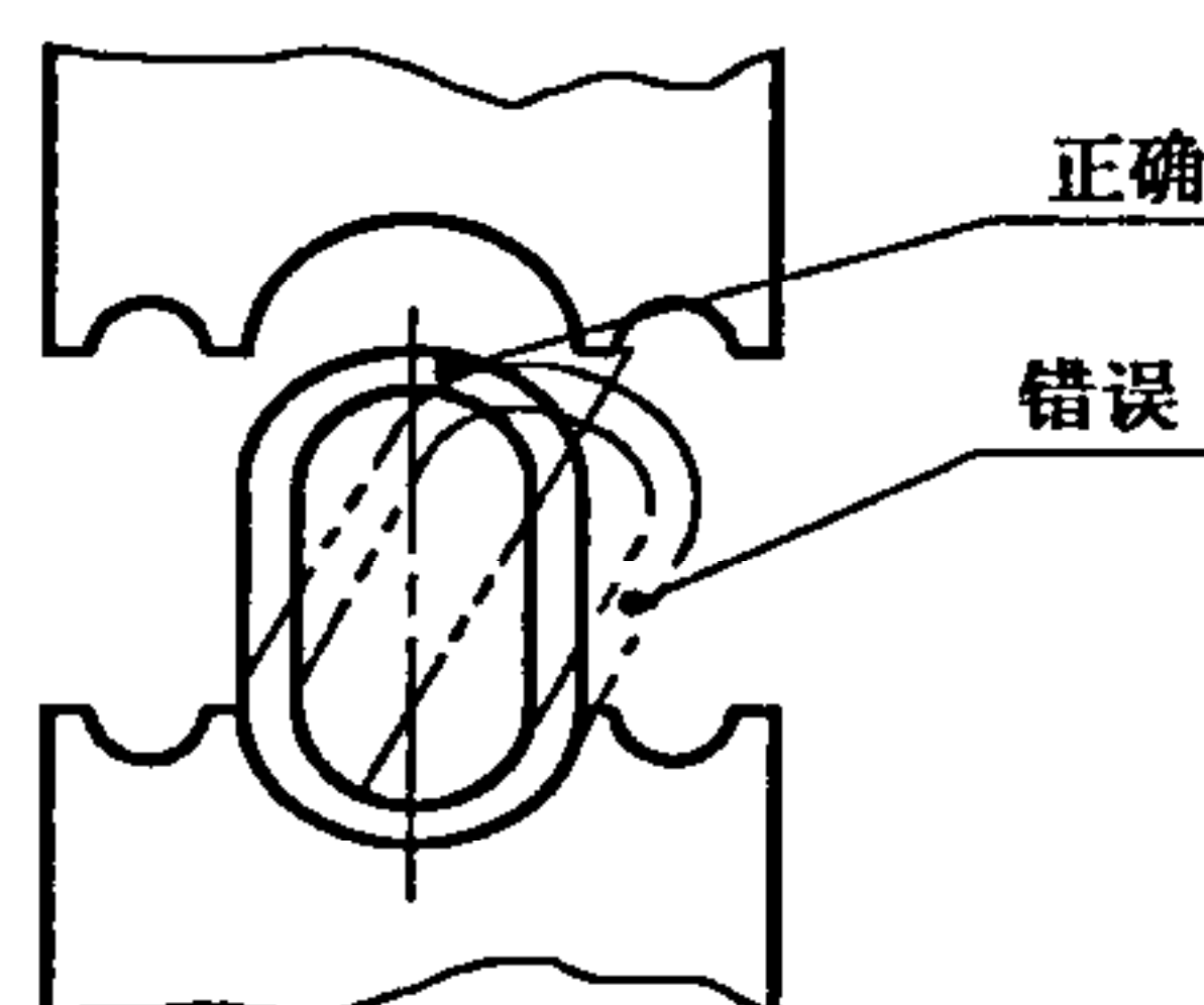
图 3 接头压制示意图
